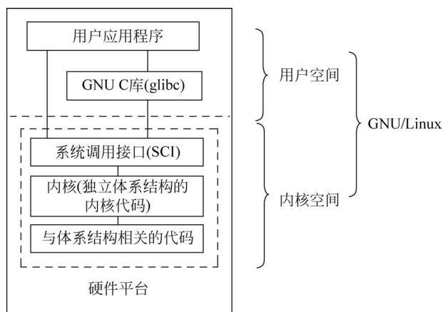
图 5-1 GNU/Linux 操作系统的基本体系结构
