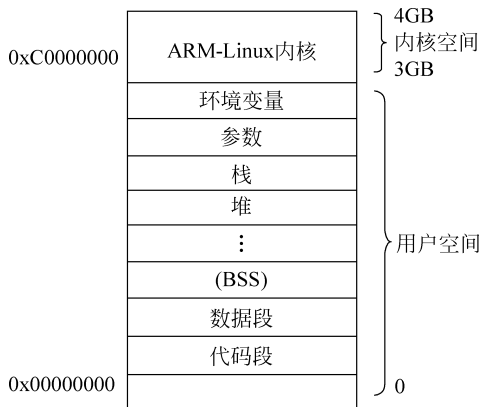
图 5-8 Linux 进程的虚拟内存空间及其组成 (32 位平台)
