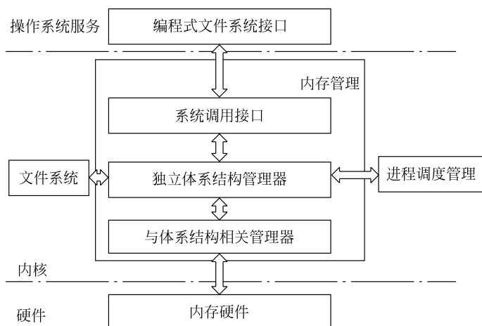
图 5-7 内存管理子系统架构
