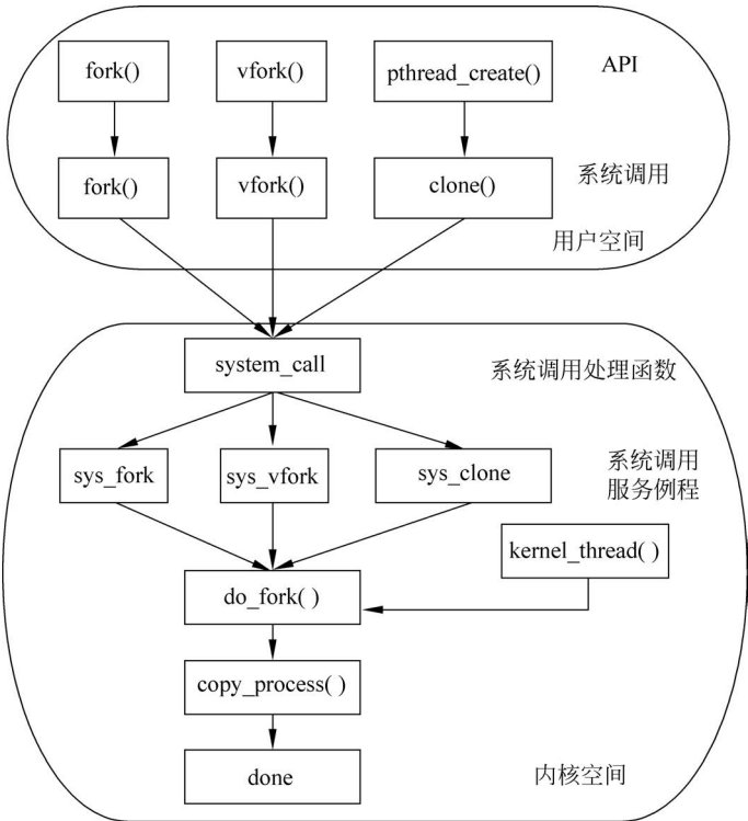
图 5-6 do_fork()函数对于进程、线程以及内核线程的应用
