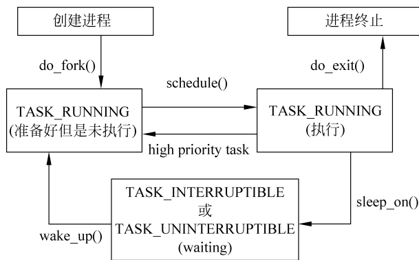
图 5-5 进程状态的切换
