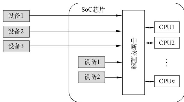
图 5-13 SMP 系统中的中断硬件组成结构
