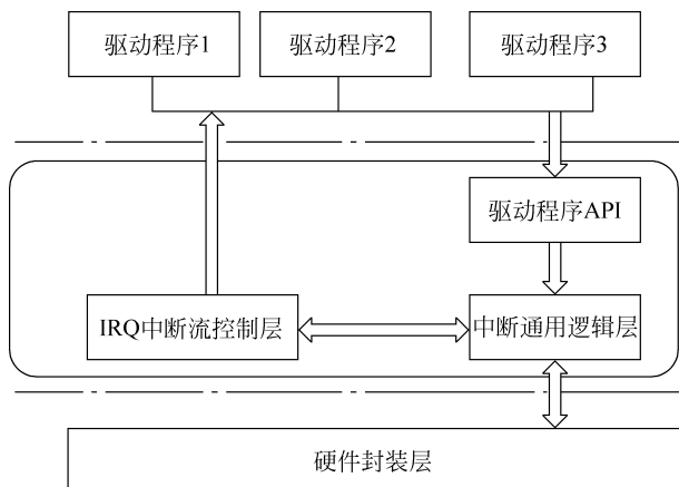
图 5-14 通用中断子系统的层次结构
