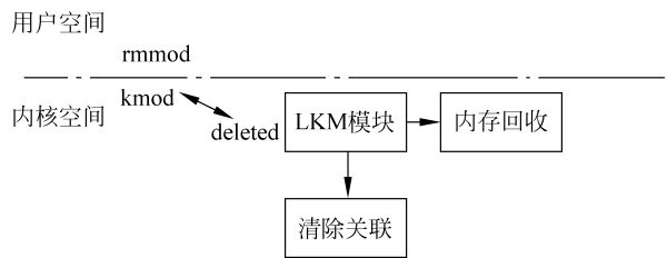
图 5-12 LKM 的卸载
