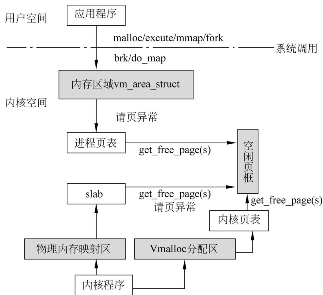
图 5-10 内核空间物理页分配技术
