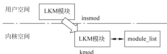
图 5-11 LKM 的加载
