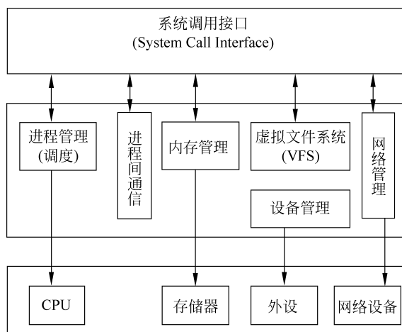
图 5-3 Linux 内核主要架构
