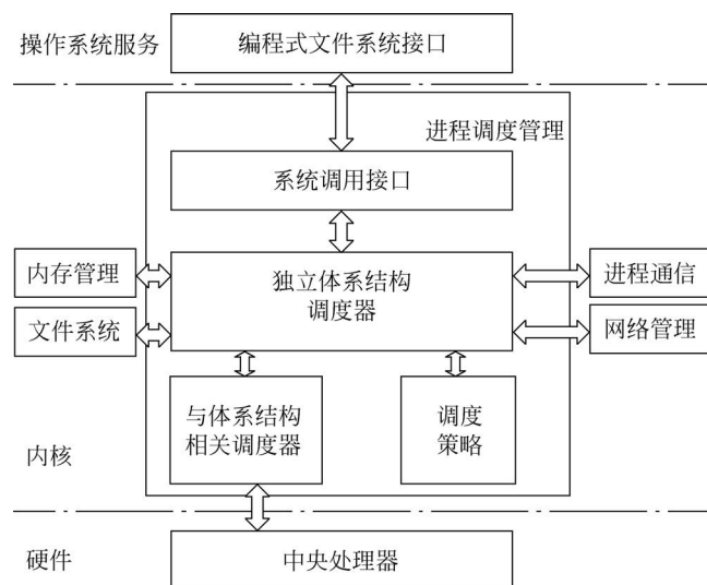
图 5-4 Linux 进程管理调度子系统基本架构
