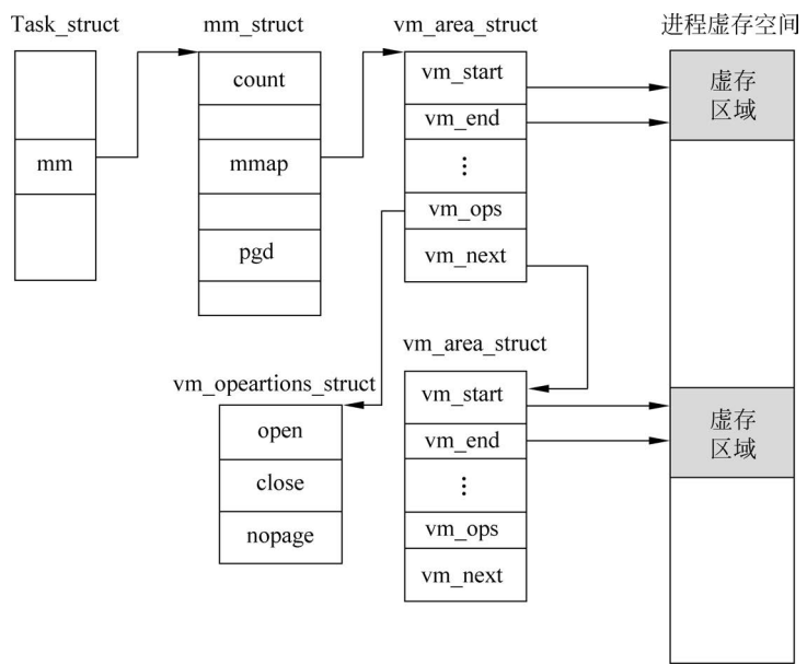
图 5-9 Linux 进程地址空间的管理模型
