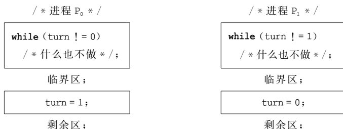
图 3-5 单标志算法
