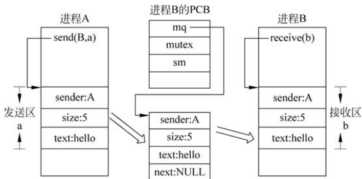
图 3-15 消息缓冲队列
