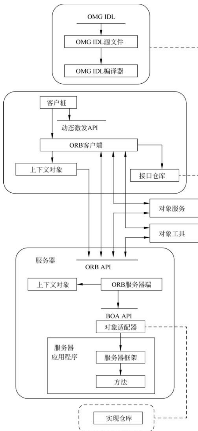
图 3-16 CORBA 的体系结构模式
