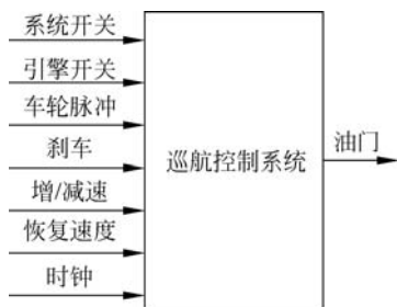
图 3-38 定速巡航控制系统简化示意图
