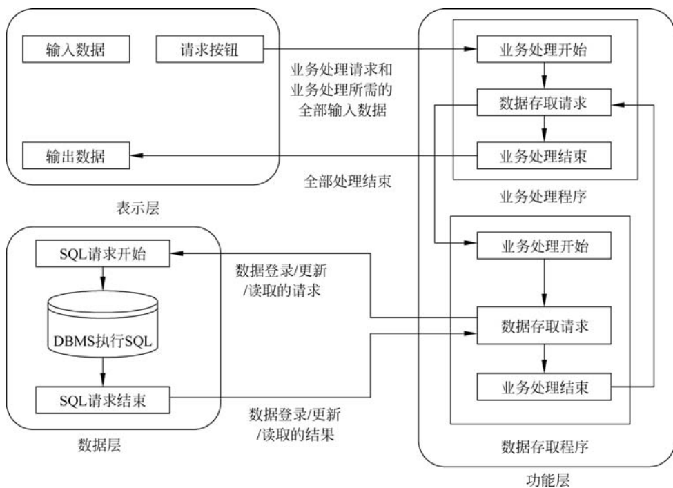
图 3-9 三层 C/S 体系结构的一般处理流程
