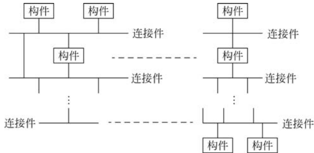
图 3-5 C2 体系结构风格
