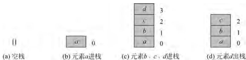
图 3.4 栈操作示意图
