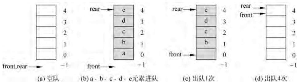
图 3.25 队列操作的示意图
