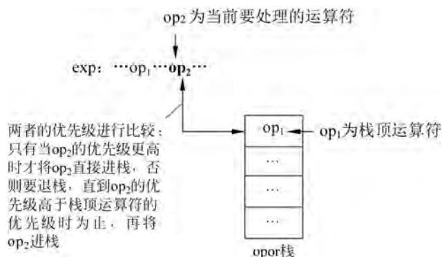
图 3.15 当前运算符的操作
