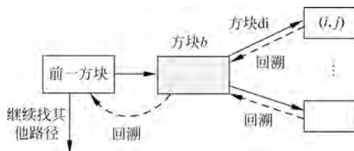
图 3.20 求迷宫路径的回溯过程
