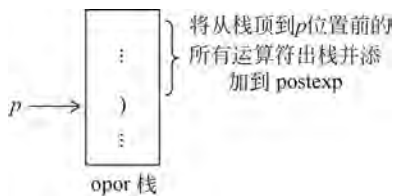
图 3.16 遇到 ')' 的处理方式
