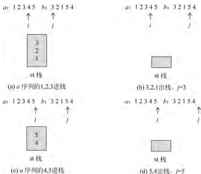
图 3.13 判断 b=[3,2,1,5,4] 是否为出栈序列的过程
