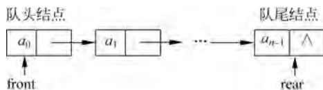
图 3.29 链队存储结构示意图
