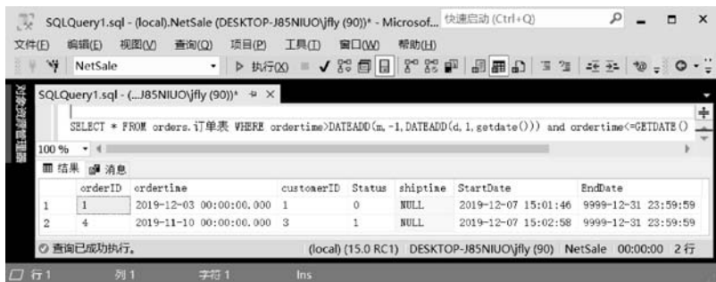
图 5-41 使用日期函数查询一个月内订单
