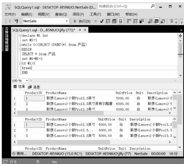
图 5-39 WHILE 循环执行结果
