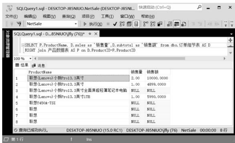
图 5-25 右连接查询结果
