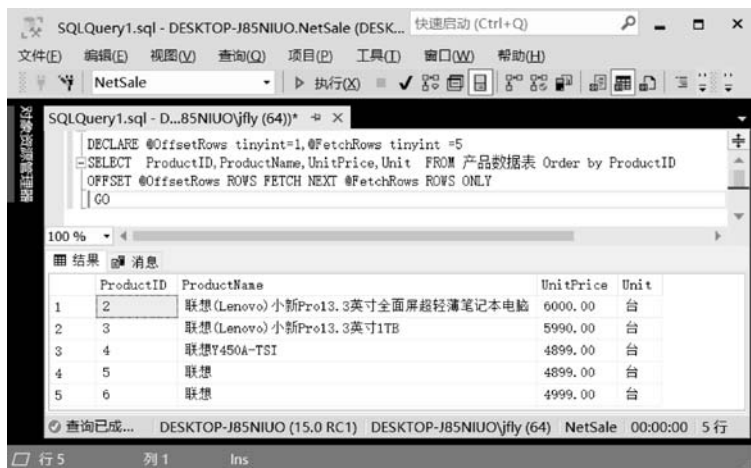
图 5-36 使用变量实现分页
