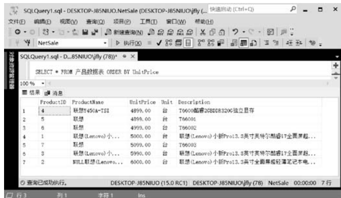
图 5-13 使用排序后的查询结果
