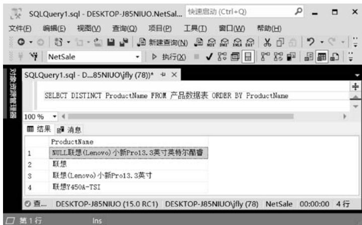
图 5-15 使用 DISTINCT 去除重复行数据
