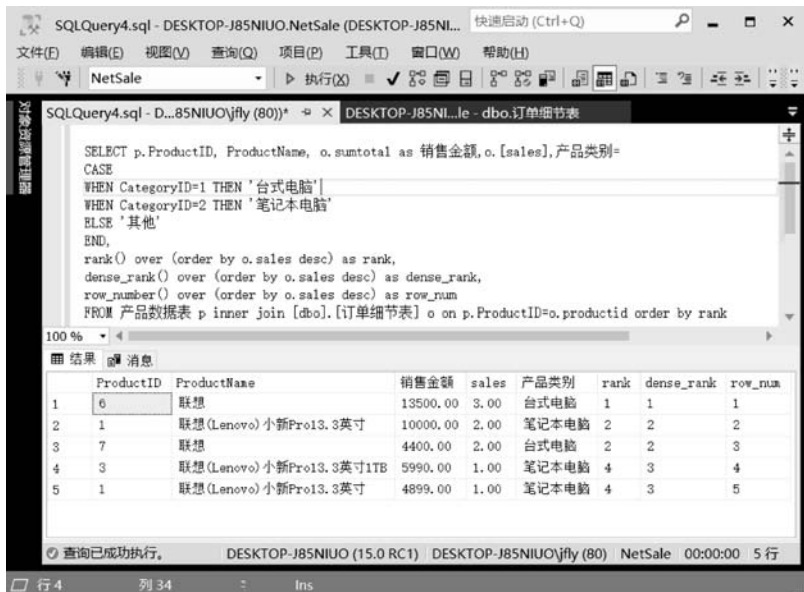
图 5-43 使用窗口函数统计销量排名
