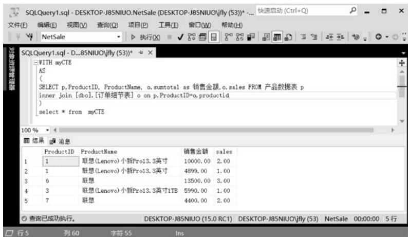
图 5-47 使用通用表表达式
