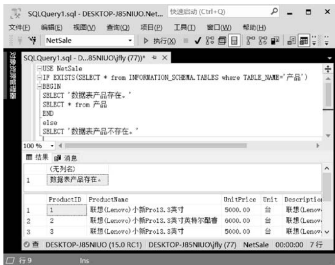
图 5-38 执行 IF…ELSE 条件分支语句
