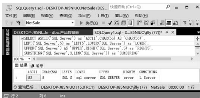
图 5-42 字符串函数执行的结果
