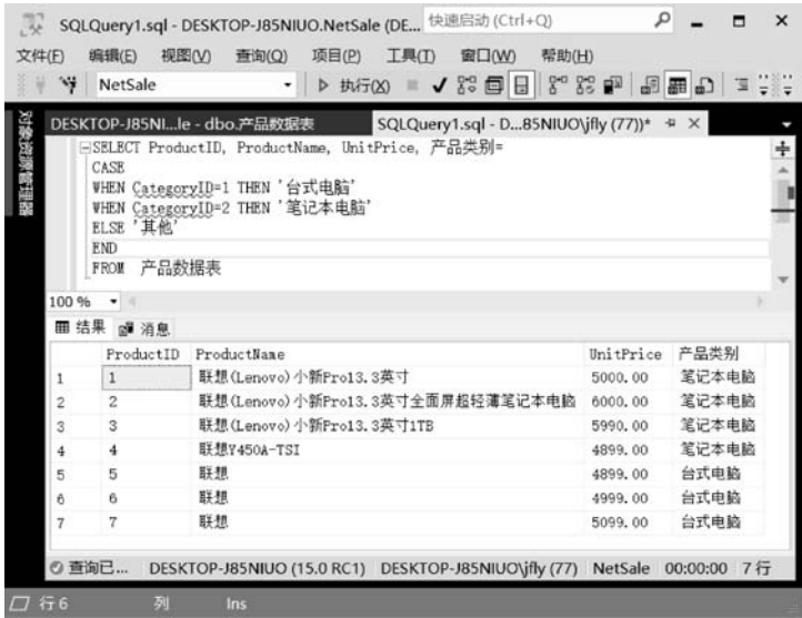
图 5-40 CASE 构造的条件分支结构执行结果
