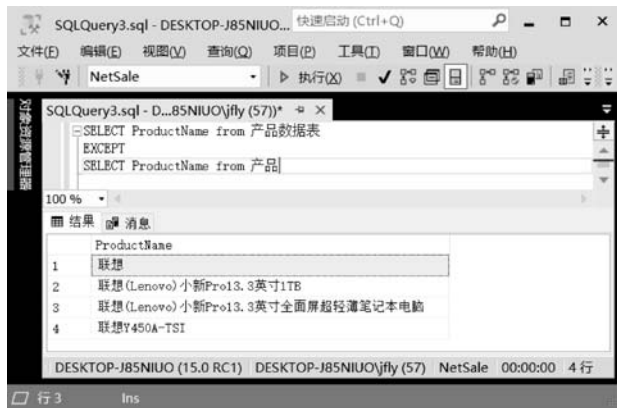
图 5-34 EXCEPT 组合查询结果
