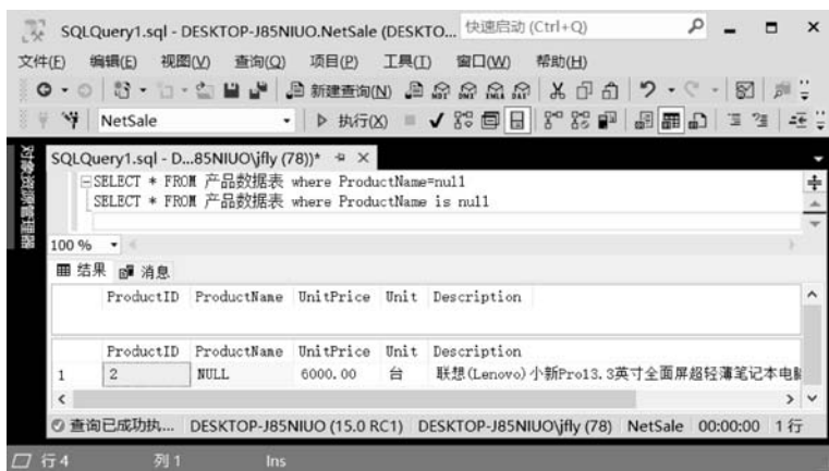
图 5-16 NULL 与 IS NULL 的区别
