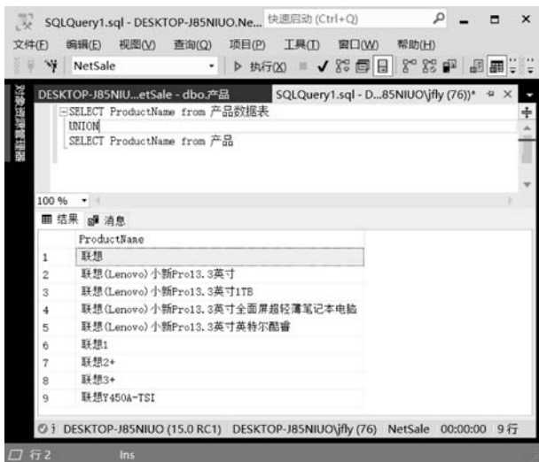
图 5-30 UNION 组合查询结果
