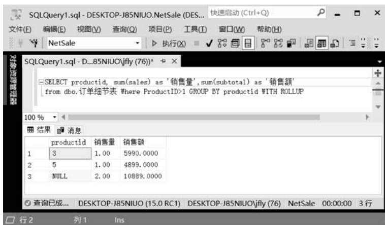
图 5-20 使用 ROLLUP 执行分组统计的结果
