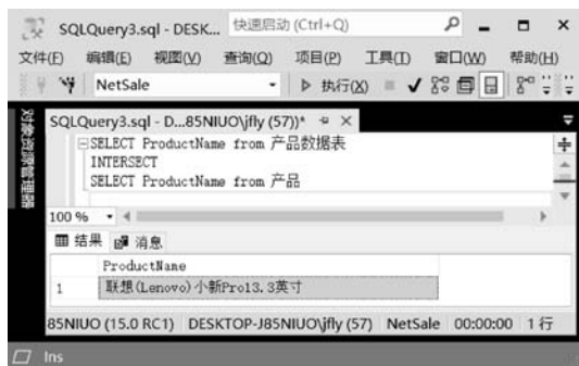
图 5-33 INTERSECT 组合查询
