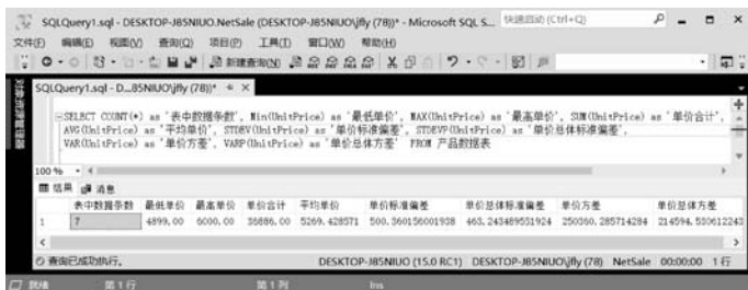
图 5-12 使用聚合函数查询的结果
