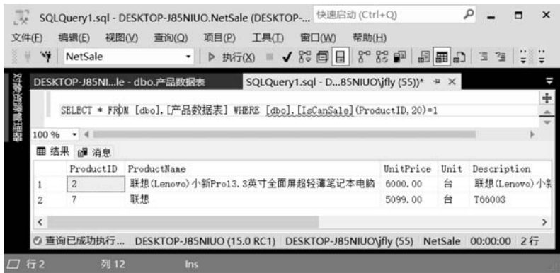
图 5-45 调用标量值用户自定义函数
