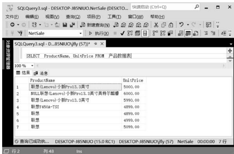
图 5-3 查询部分列的数据
