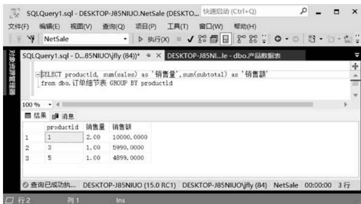
图 5-18 使用 GROUP BY 分组统计
