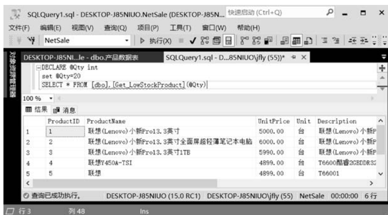
图 5-46 调用表值函数
