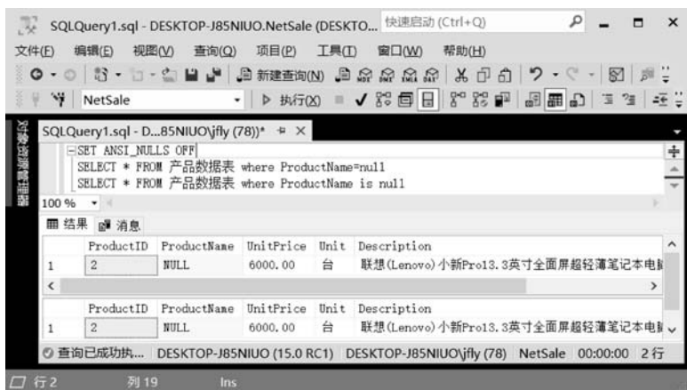
图 5-17 设置 SET ANSI_NULLS OFF 后 NULL 与 IS NULL 相同
