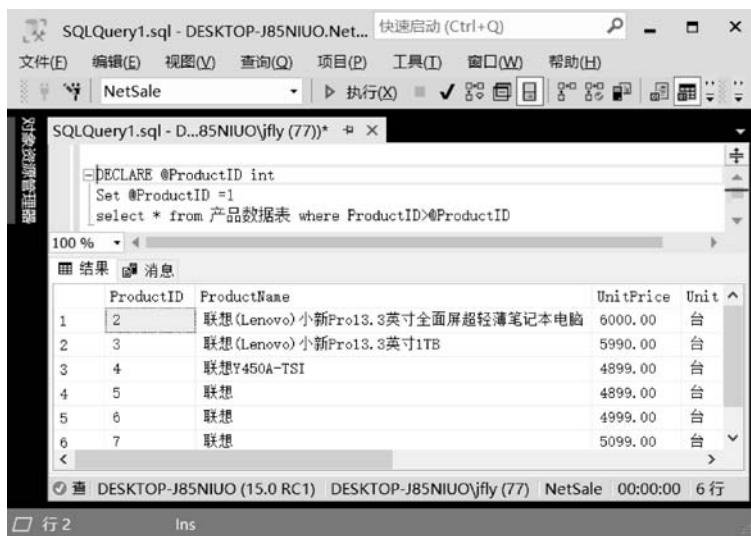
图 5-37 使用变量
