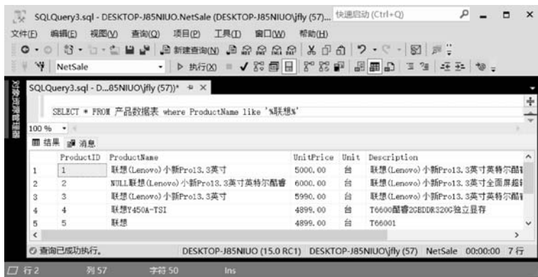
图 5-7 模糊查询的结果
