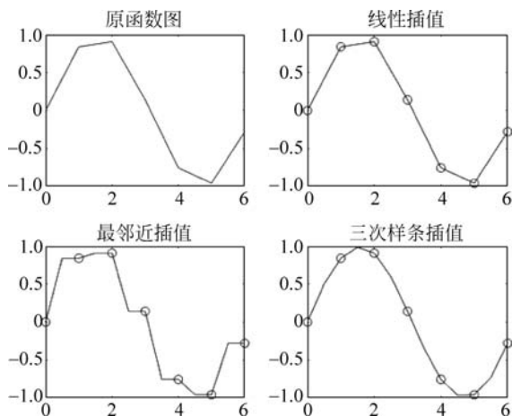
图 3.10 三种插值与原函数图的比较
