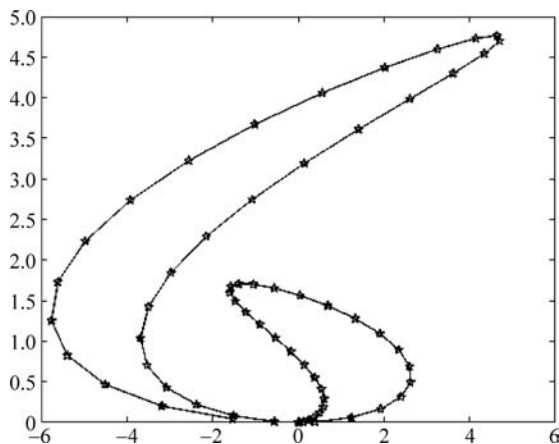
图 3.2 例 3-24 函数曲线
