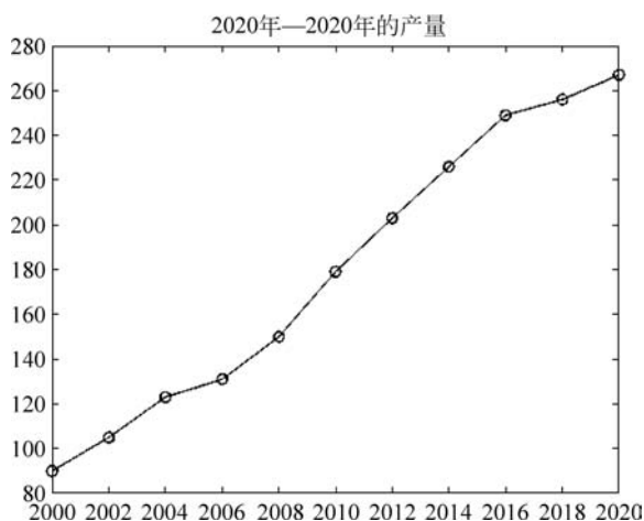
图 3.12 默认插值曲线
