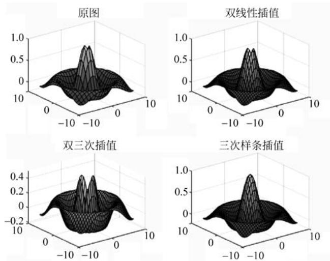
图 3.14 四种插值曲面拟合结果
