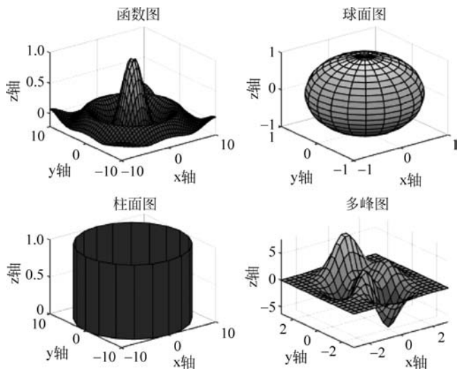
图 3.8 例 3-30 函数图像
