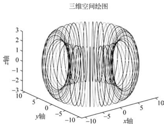
图 3.5 三维空间曲面图
