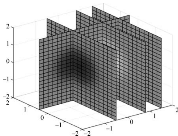
图 3.9 三维切片图
