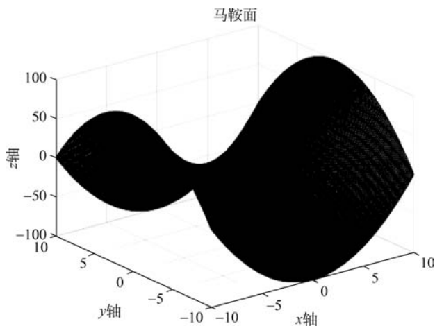
图 3.7 三维曲面图
