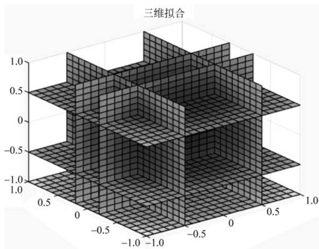
图 3.15 三维插值图
