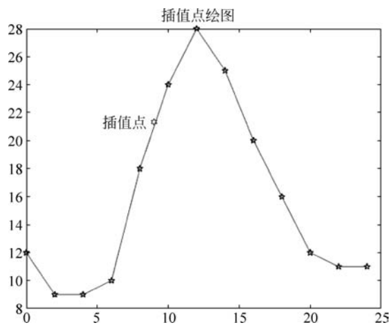
图 3.11 插值绘图
