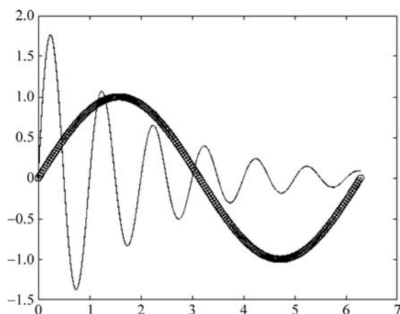
图 3.1 例 3-23 函数曲线
