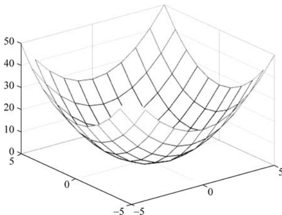
图 3.6 三维网格曲面图
