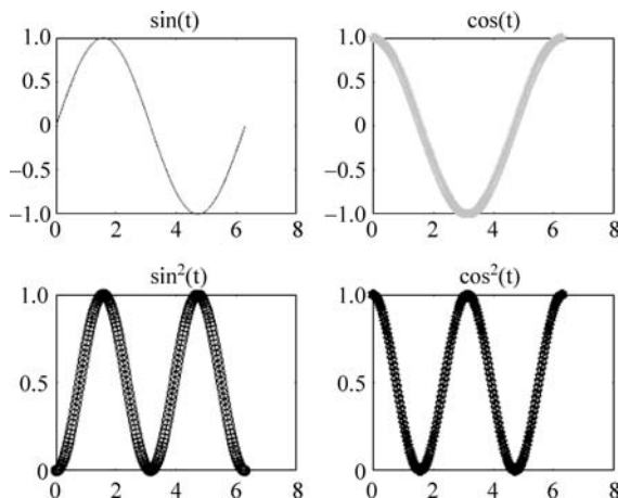
图 3.4 绘制子图
