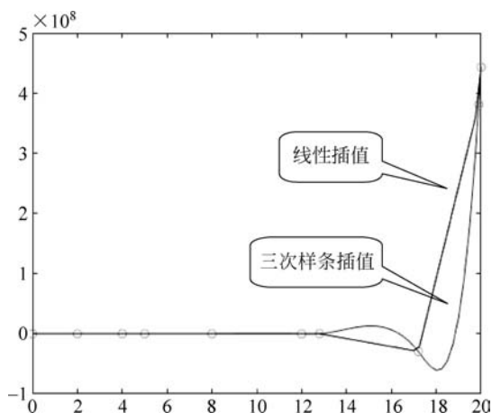
图 3.13 三次样条插值与线性插值绘图
