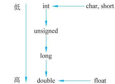
图 3-3 混合运算的数据类型转换规则
