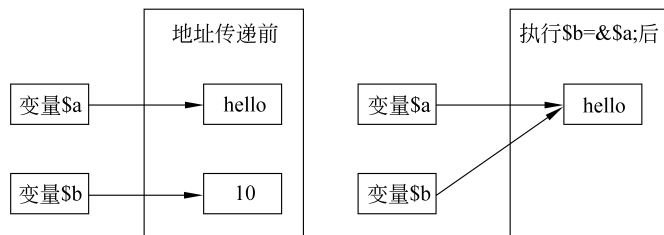
图 3-2 引用赋值——变量地址传递示意图
