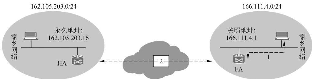
图 5-7 外部代理的工作原理
