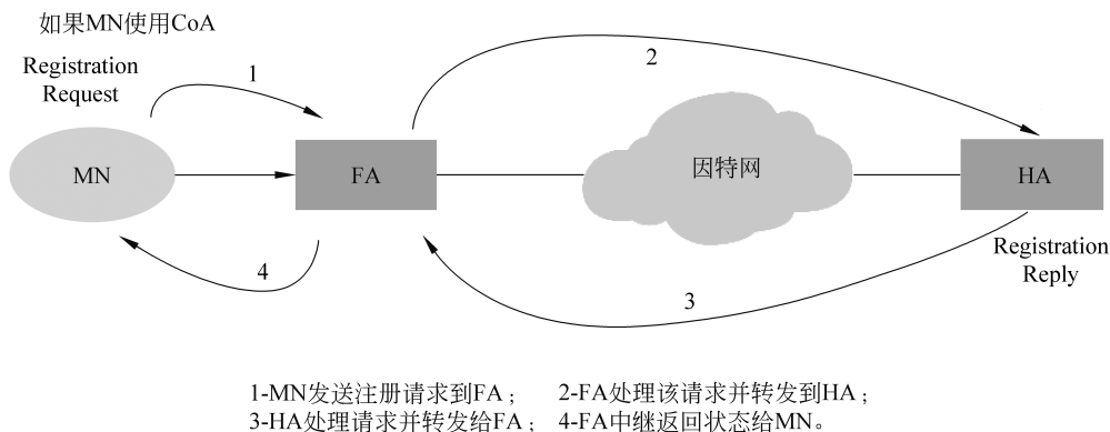
图 5-9 通过外部代理发送注册请求示意图
