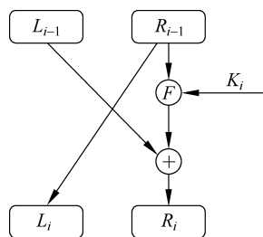
图 3.6 DES 每轮结构
