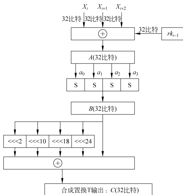
图 3.34 合成置换 T
