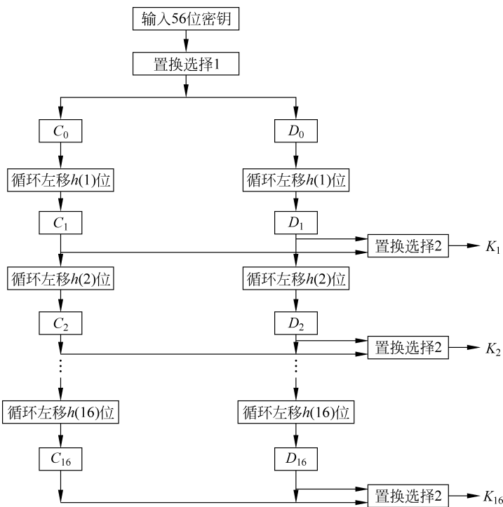
图 3.13 子密钥的产生过程
