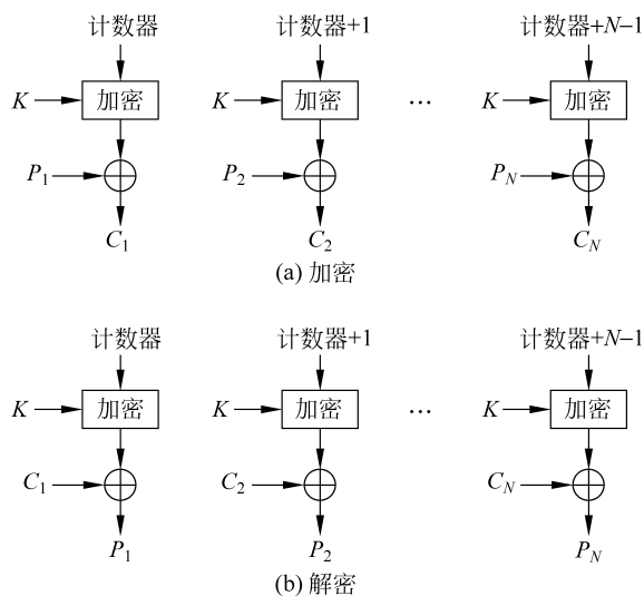
图 3.51 计数器模式
