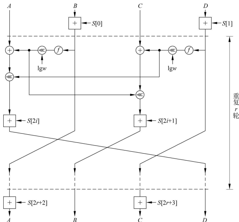
图 3.37 RC6 的加密过程
