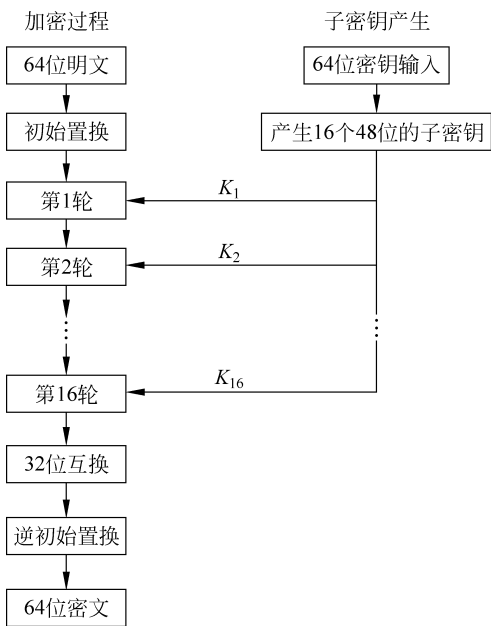
图 3.4 DES 加密算法简图
