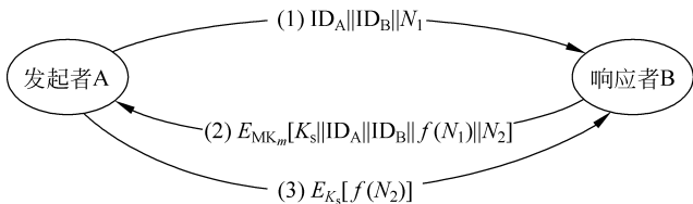
图 3.57 无中心的密钥分配过程
