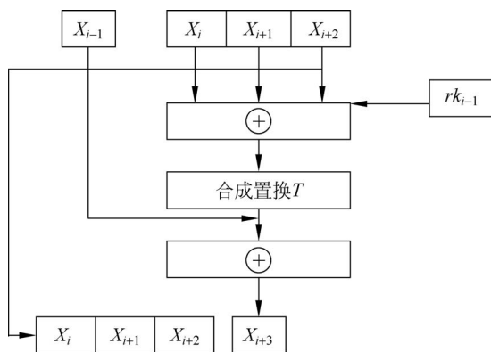
图 3.33 SM4 加密每轮的结构
