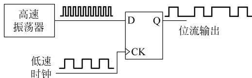
图 3.53 振荡采样随机数发生器
