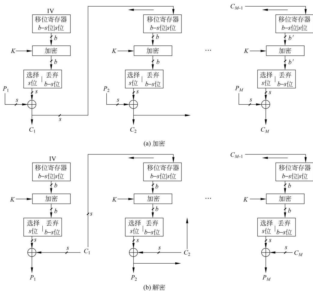
图 3.49 密码反馈模式
