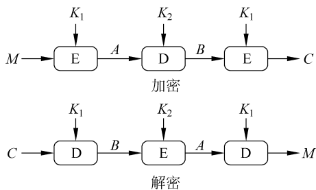
图 3.18 三重 DES
