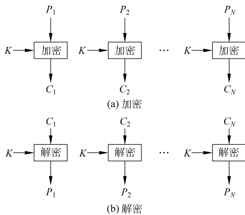
图 3.47 电子密码本模式
