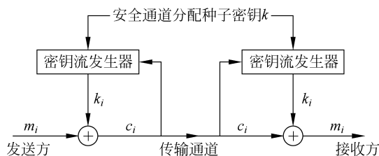
图 3.43 自同步流密码
