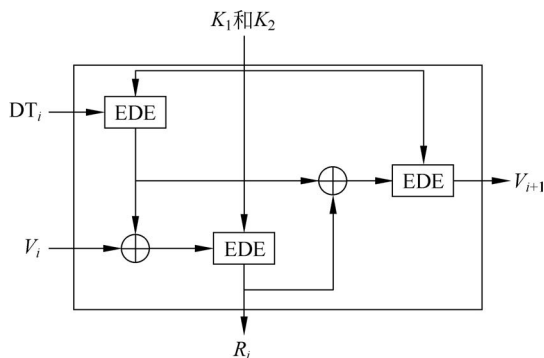
图 3.55 ANSI X9.17 伪随机数生成器
