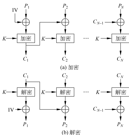
图 3.48 密码分组链接模式
