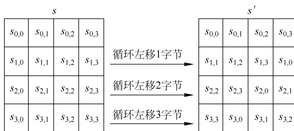
图 3.26 对 State 的各行移位
