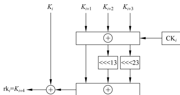
图 3.36 SM4 轮密钥生成
