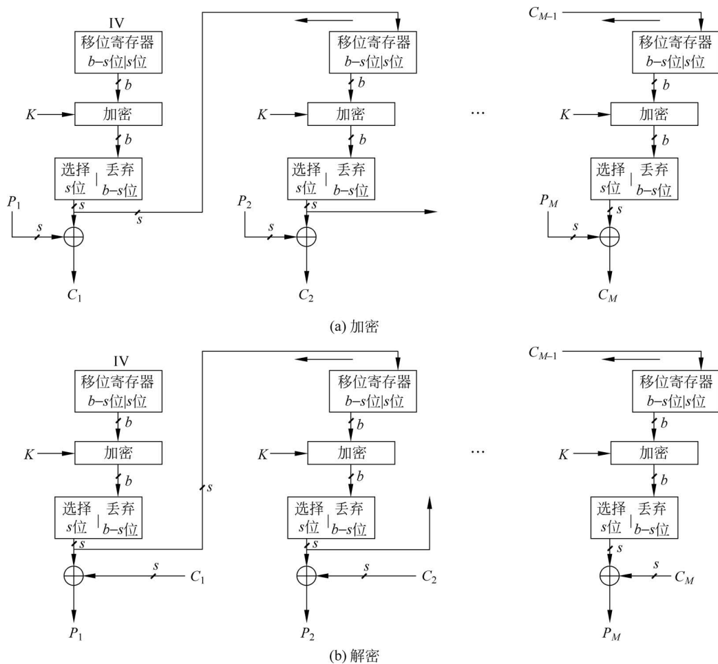
图 3.50 输出反馈模式
