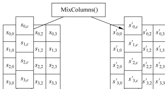
图 3.27 列混淆变换示意图
