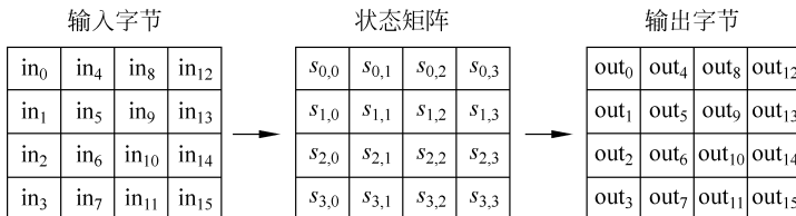
图 3.22 状态矩阵、输入和输出
