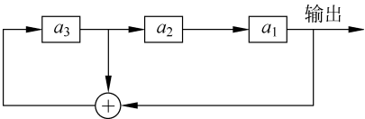
图 3.46 一个三级移位寄存器
