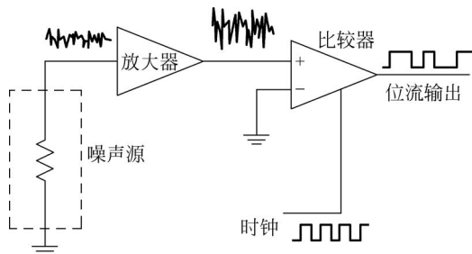
图 3.52 利用热噪声的随机数发生器
