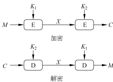
图 3.17 双重 DES
