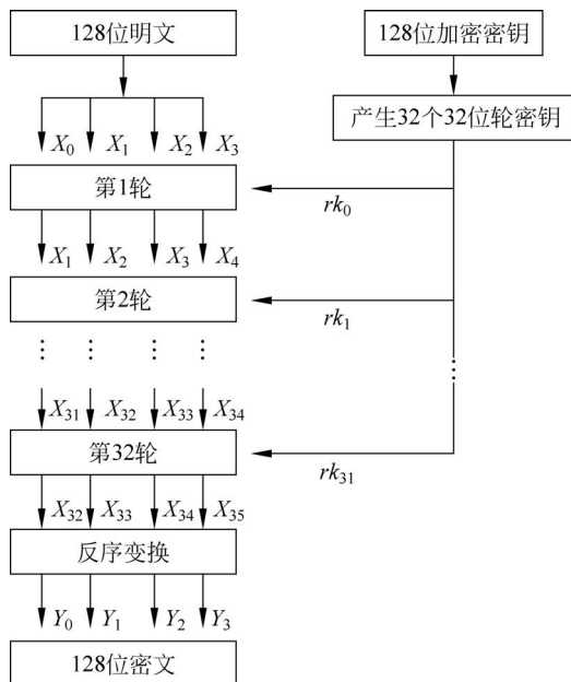
图 3.32 SM4 加密过程
