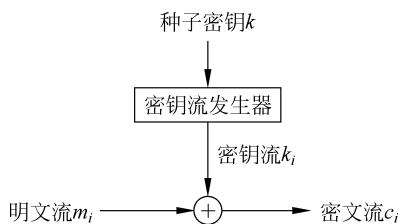
图 3.41 流密码加密过程
