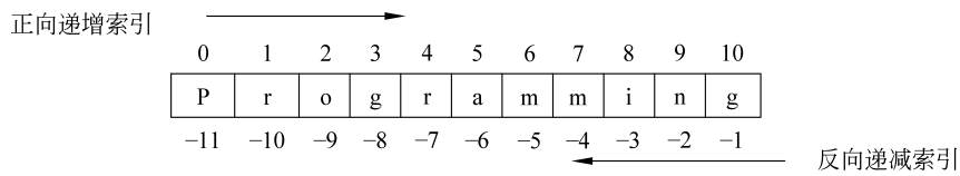
图 3-1 字符串索引
